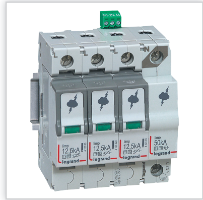
Ograniczniki przepięć ON300 – typ 1 (klasa B), typ 2 (klasa C), typ 1+2 (klasa B+C); poziom ochrony do 1,2 kV; rozwiązania 1P, 1P+N, 2P, 3P, 3P+N i 4P; wymienne wkłady do ochronników.
